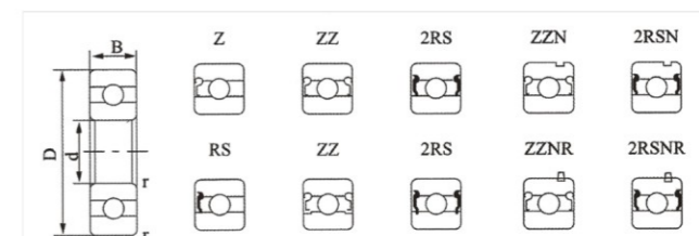
型号/Model: 604-609、6000-6022 规格/Spec: ZZ、Z、2RS、RS、OPEN、NR、2RSL
